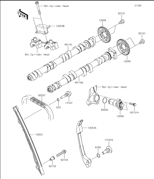
7 Camshaft(s)/Tensioner
