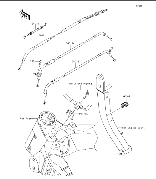
51 Cables
