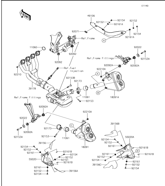
5 Muffler(s)
